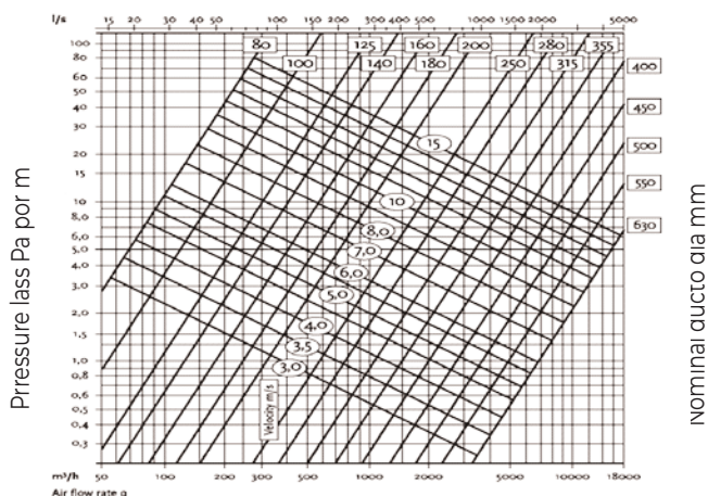
Pérdida de presión conducto recto
